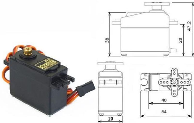
Рис. 1. Сервопривод
